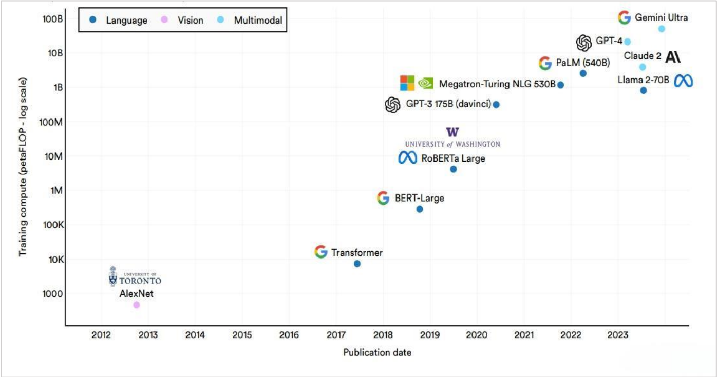
2012年-2023年各领域著名人工智能大模型训练计算量
