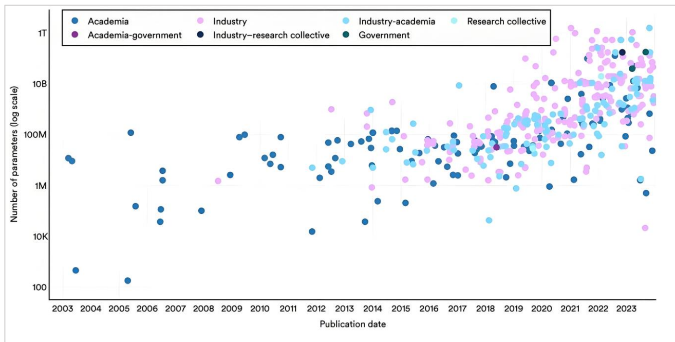
2003年-2023年主要人工智能大模型参数数量
