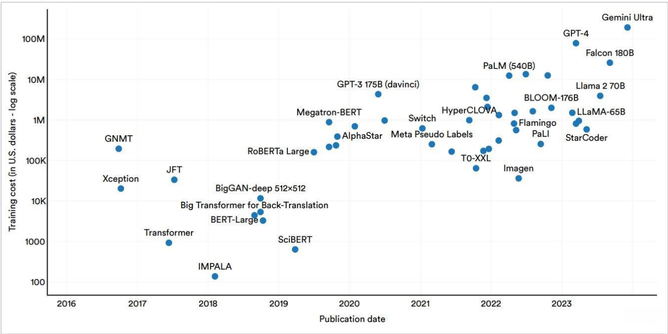
2016-23年部分AI模型的训练成本估算
