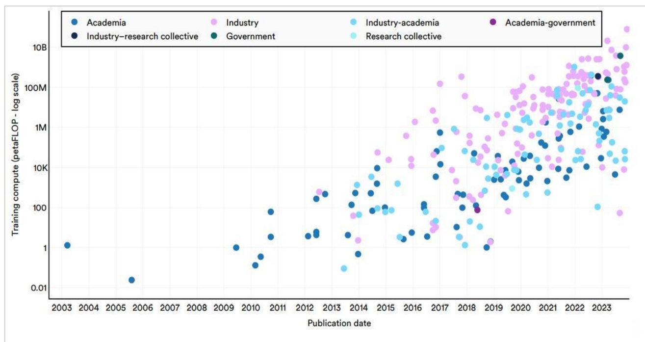
2003年-2023年主要人工智能大模型训练算力需求
