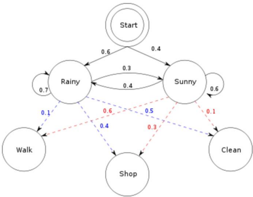
HMM模型示意图
